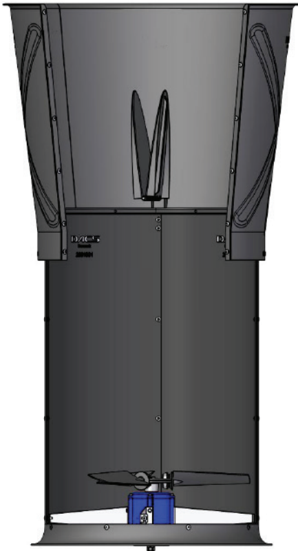
Обратный клапан (бабочка)
